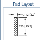
DWG. 1 MATERIAL: .008 (.20) Brass
