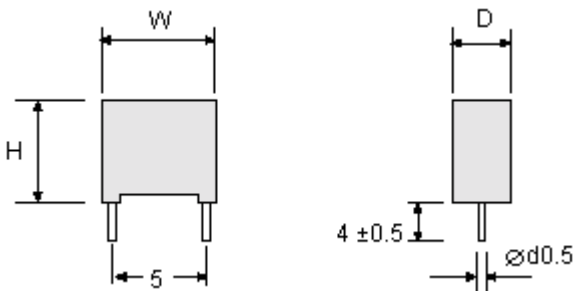
Dimensions : Millimetres
